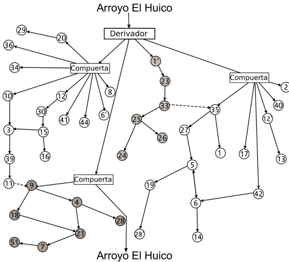
Figura 12. Flujo de agua en el sistema de boleos de GME
